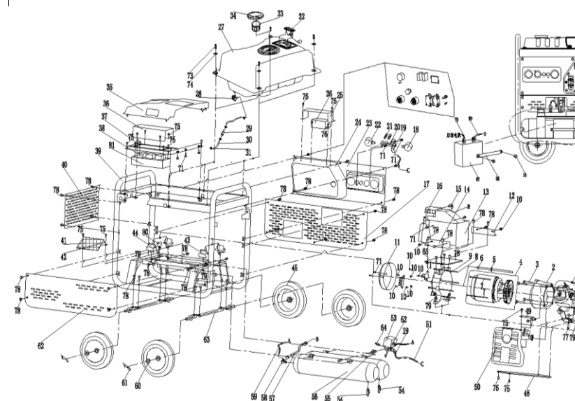
10002-00068-00 5KW三合一工频焊机 MULTIPLWX 9600RS/D8款 整机爆炸图
